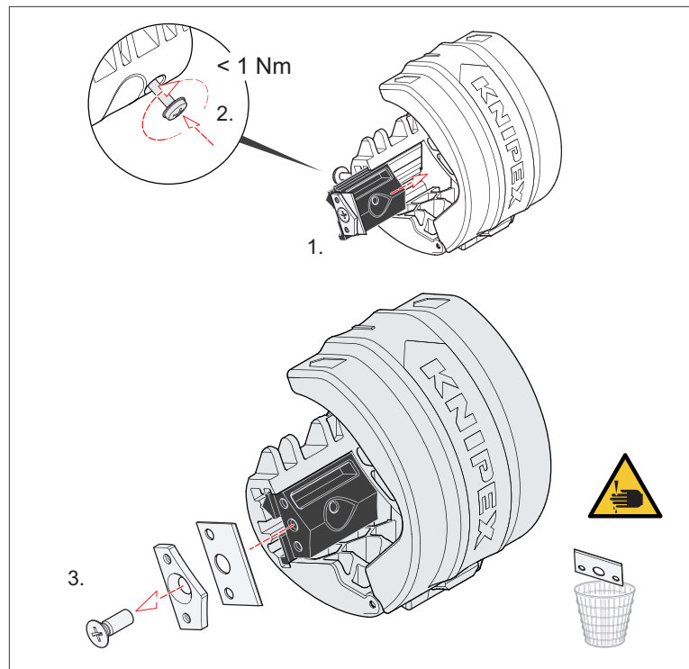
Klinge ausbauen
